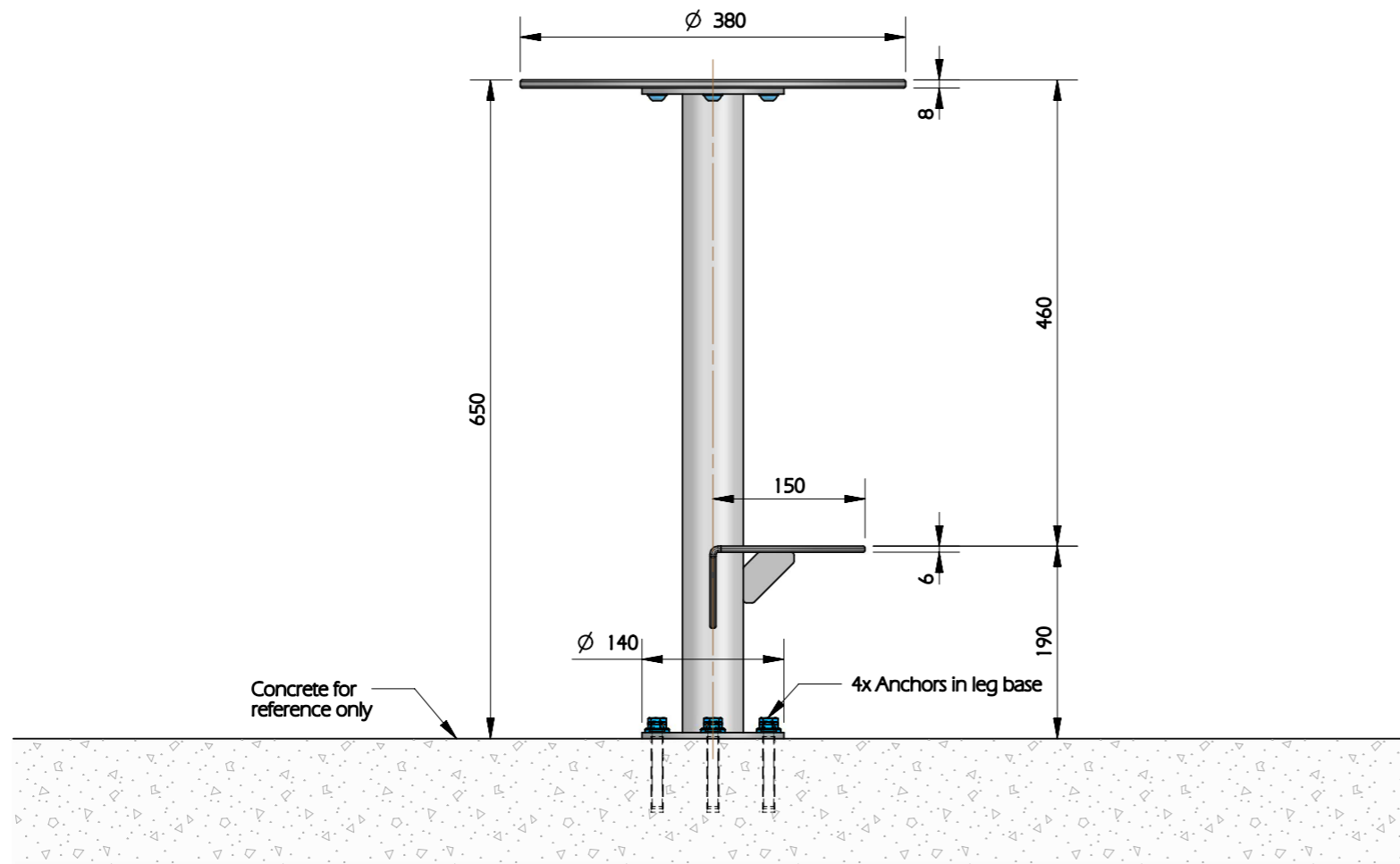
ELEVATION
