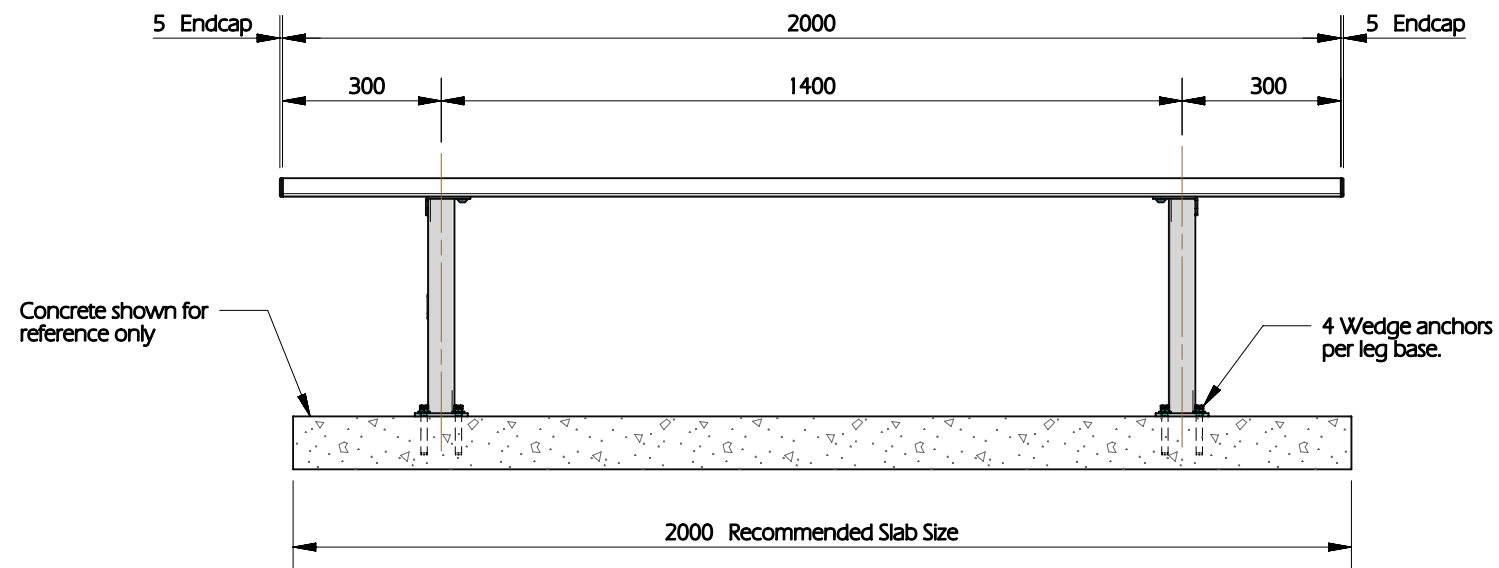
ELEVATION
