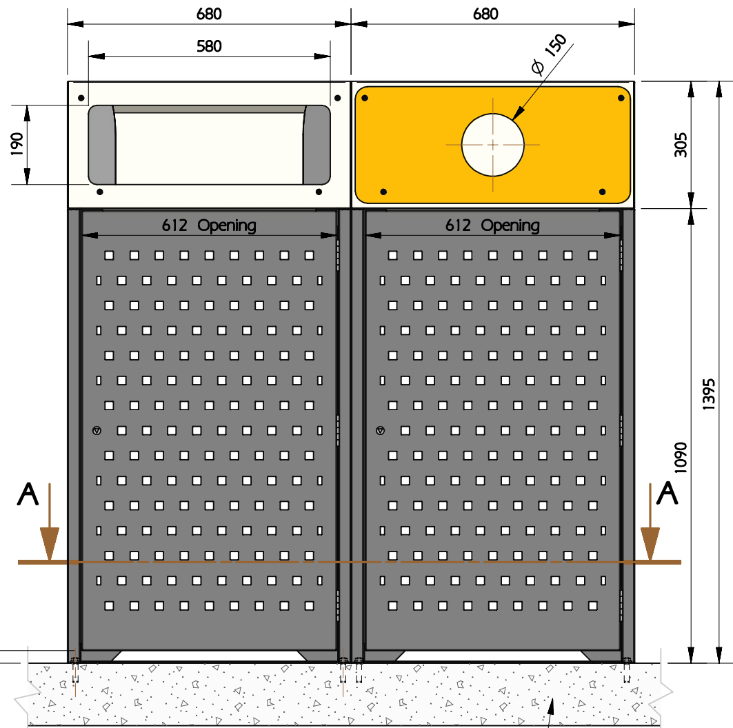
ELEVATION SCALE: NTS
