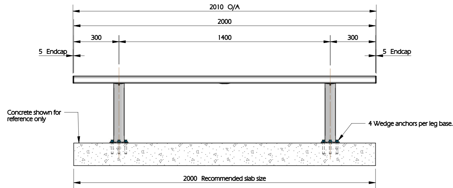
ELEVATION
